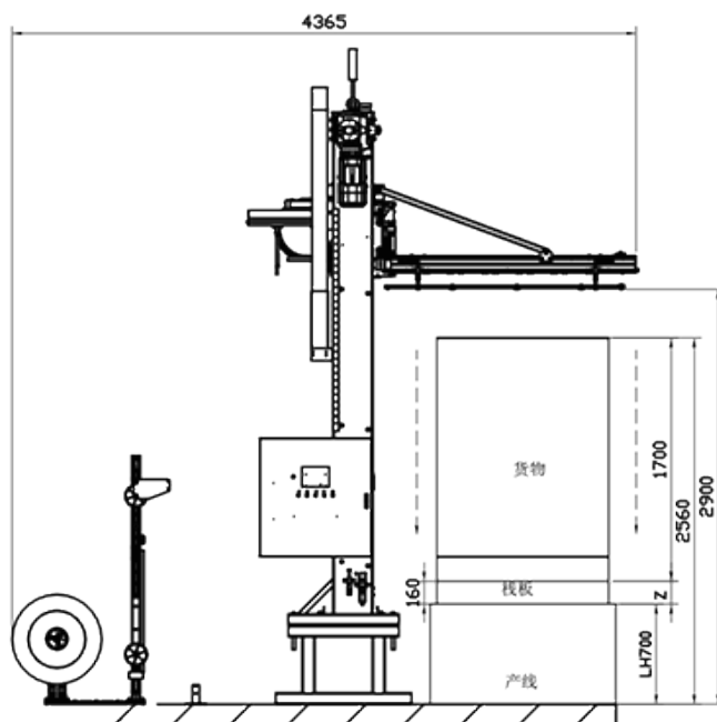
侧视图
