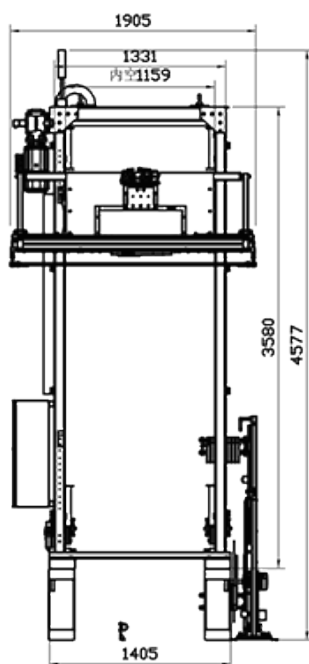
正视图
